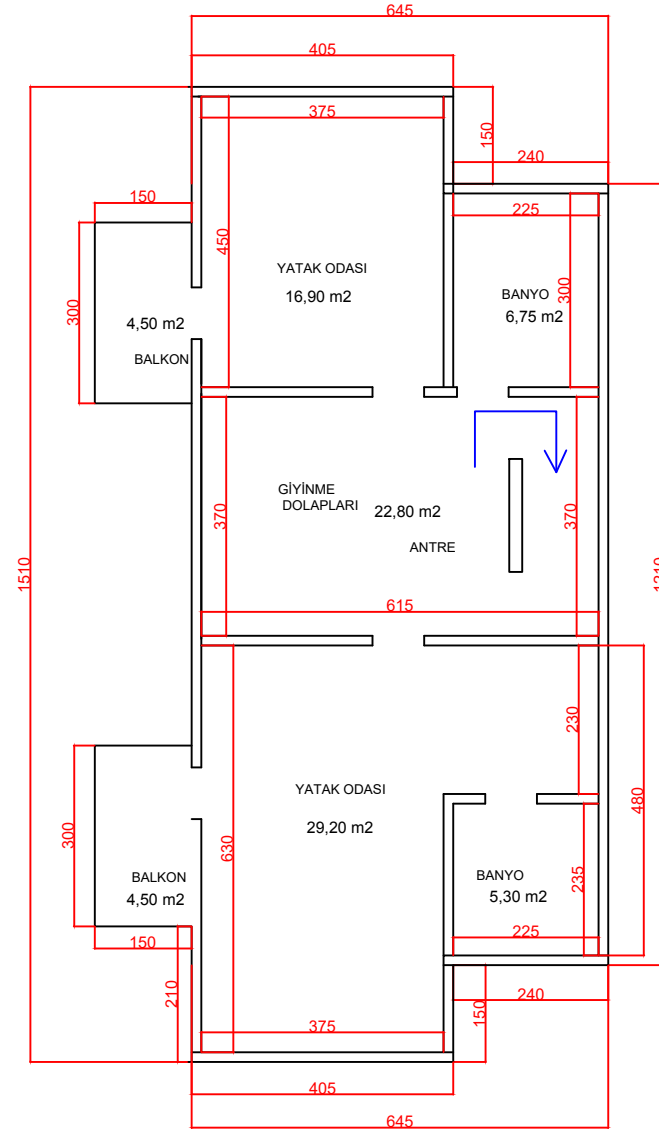
1 KAT PLANI Brüt : 100 m²
