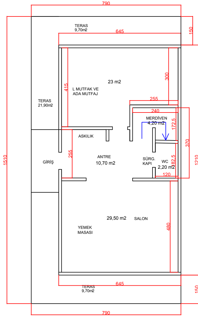
ZEMİN KAT PLANI Brüt : 120 m²
