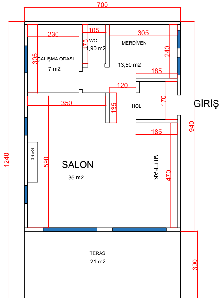
ZEMİN KAT PLANI Brüt :87 m2
