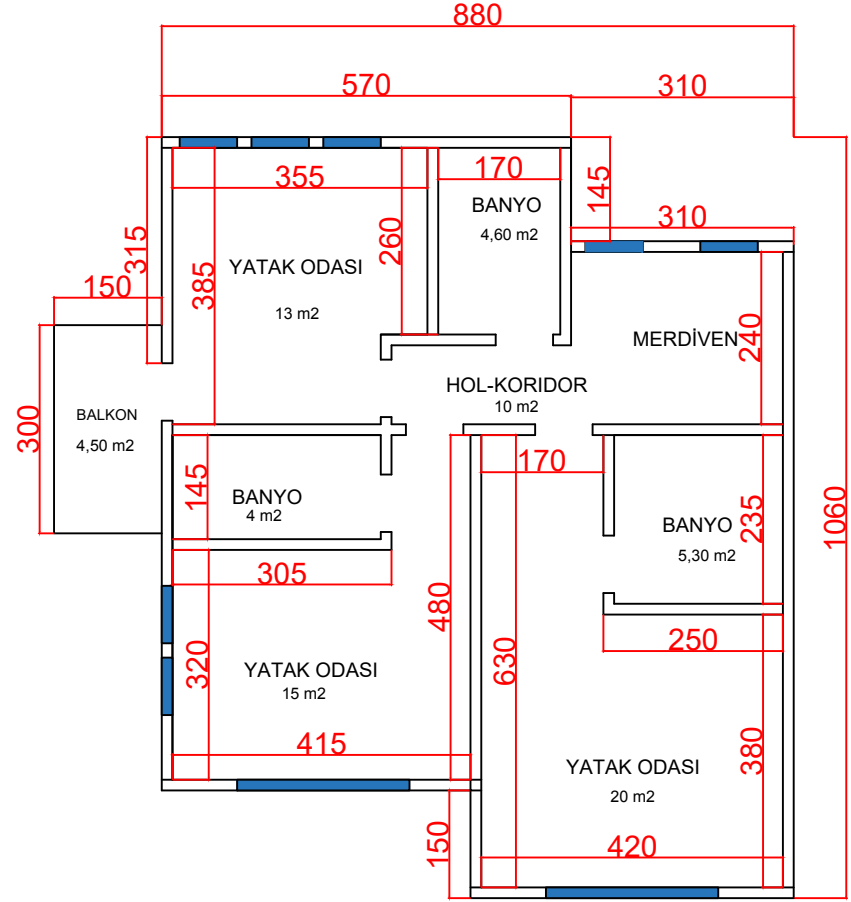
1. KAT PLANI Brüt : 87 m2
