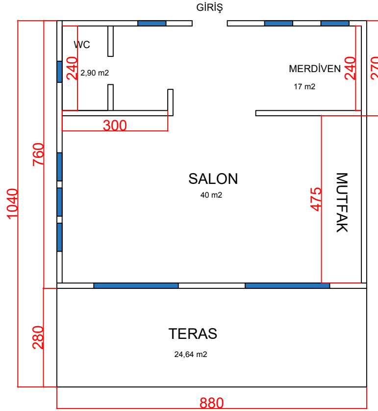
ZEMİN KAT PLANI Brüt : 92 m2
